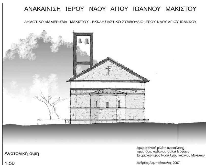
Ανατολική όψη
