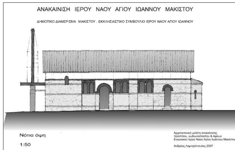
Νότια όψη
